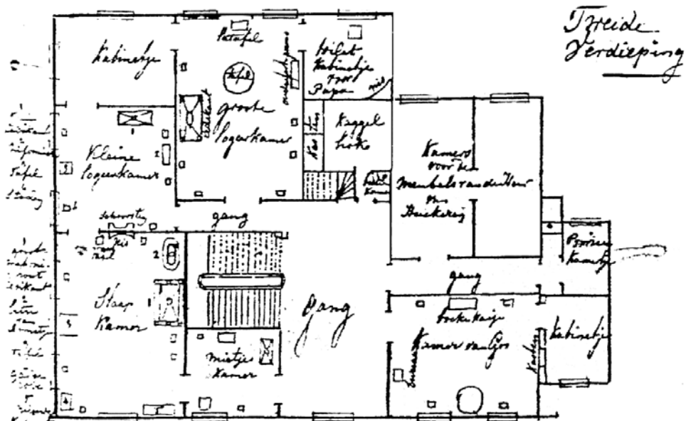
Plattegronden van de begane grond en de verdieping van De Cloese uit 1821
