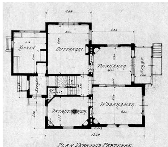
Boven de Plattegrond van de ambtswoning van Artis, 1897, collectie NAI /klix-22, onder de plattegrond van de middelste villa aan de Nieuweweg in Lochem, 1884.
